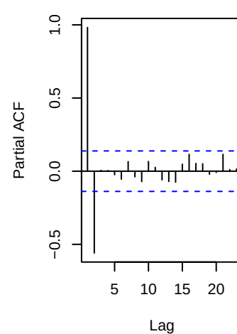
ARIMA(1,1,0) PACF
