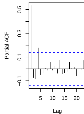
ARIMA(1,1,0) PACF
